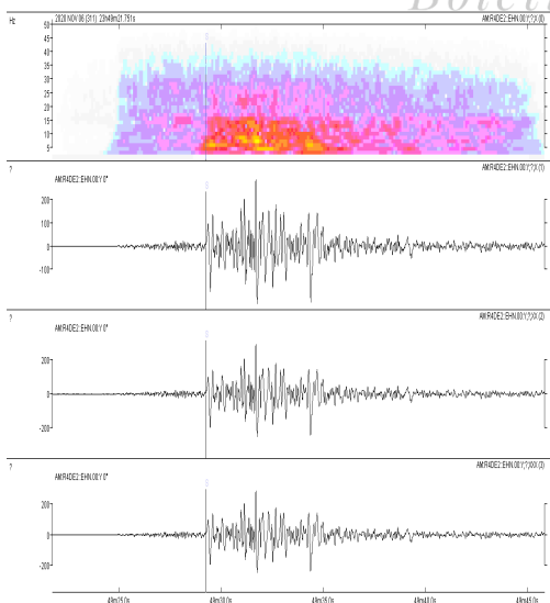
Figura 5. Sismograma y espectrograma del evento sísmico ocurrido el día 06-11-2020 a las 23:49 (UTC).
