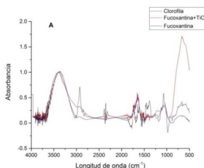
Figura 2. Espectro FTIR para muestras de clorofila (negro), fucoxantina (azul) y fucoxantina adsorbida en TiO 2 (rojo), al 1%.
