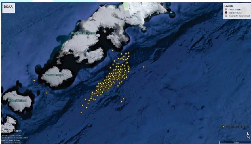
Figura 4. Distribución de los eventos sísmicos (periodo 26 de agosto al 11 de septiembre) localizados.
