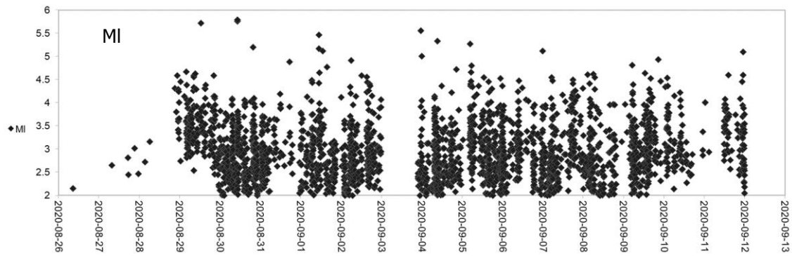
Figura 3. Distribución de las magnitudes respecto a las fechas (periodo 26 de agosto a 11 de septiembre).
