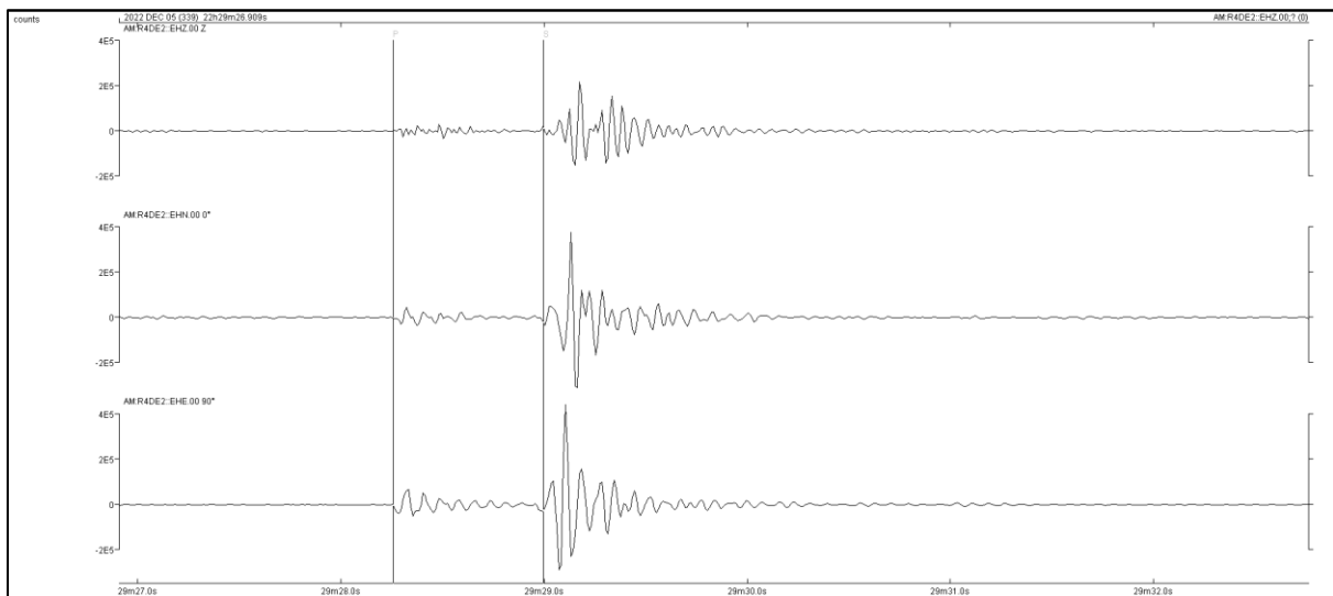
Figura 1. Forma de onda de los eventos sísmicos ocurridos el día 05 de diciembre del 2022.
