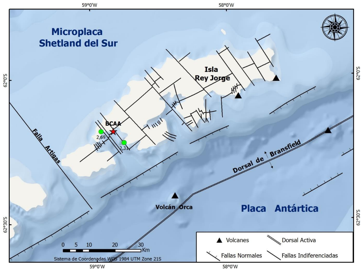
Figura 2. Localización de los eventos sísmicos ocurridos el día 05-12-2022.
