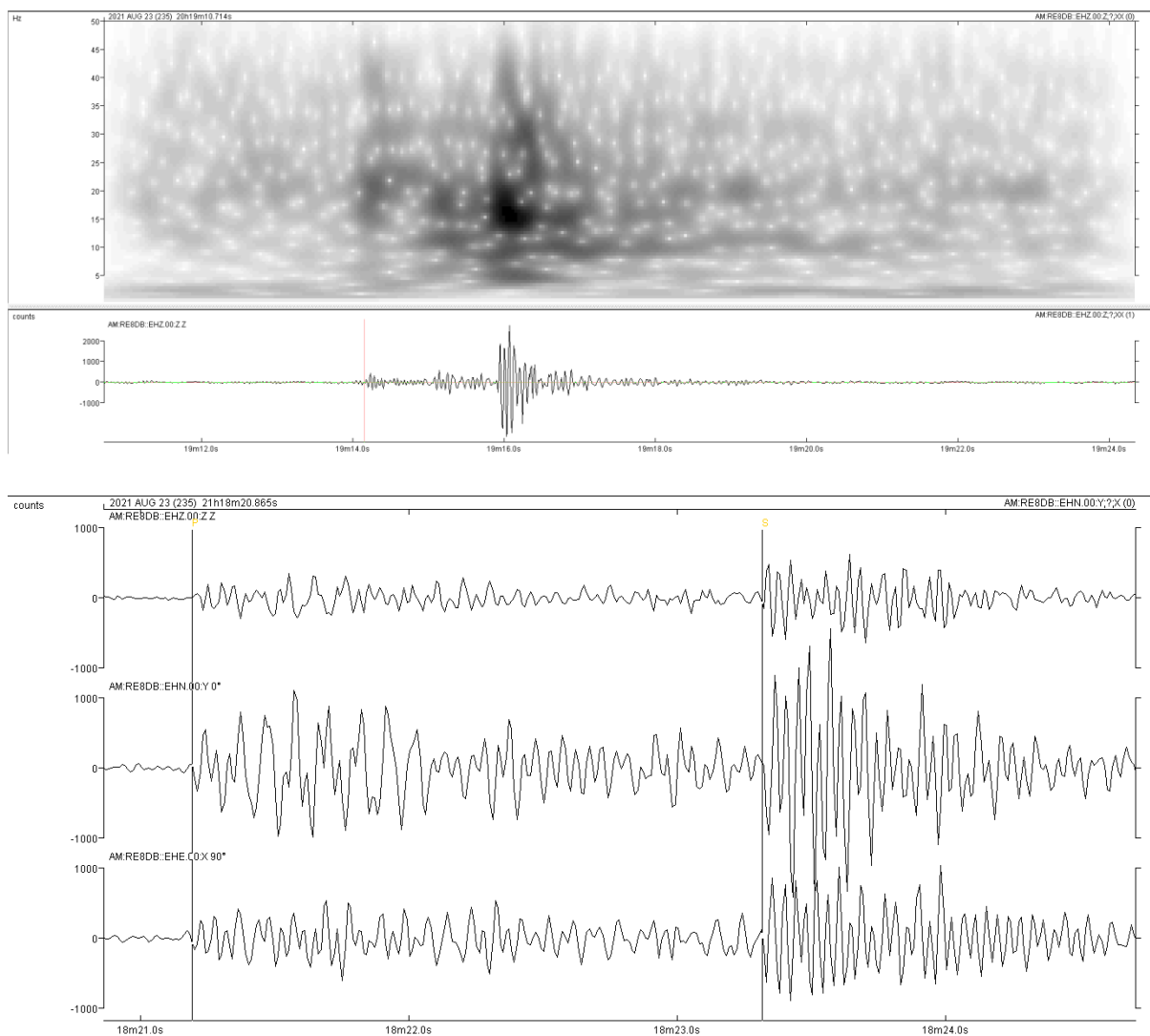
Figura 1. Trazas sísmicas para la estación en las que se detectaron los eventos. A) evento ocurrido a las 20:19 H (UTC), B) evento ocurrido a las 21:18 H (UTC)
