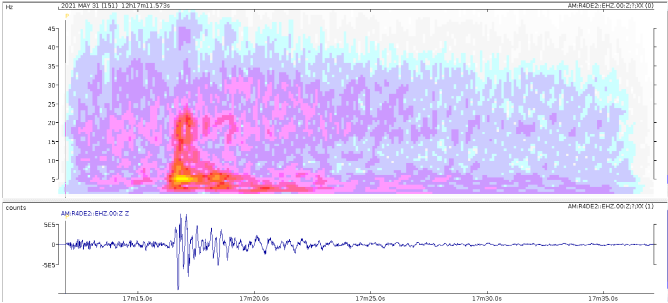
Figura 2. Forma de onda de eventos del evento del día 31/05/2021 (12:17 ) de M_{Lz} = 4.79 .
